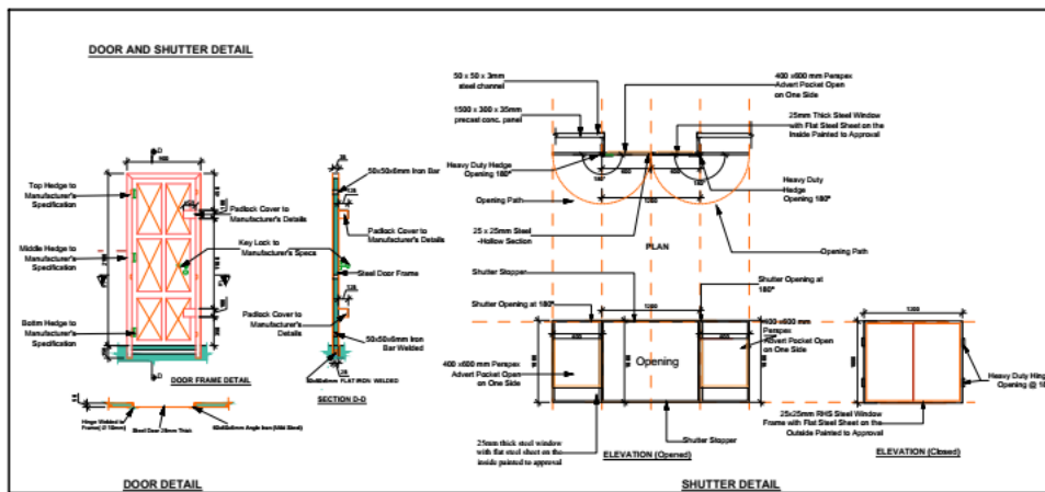
DOOR DETAIL
