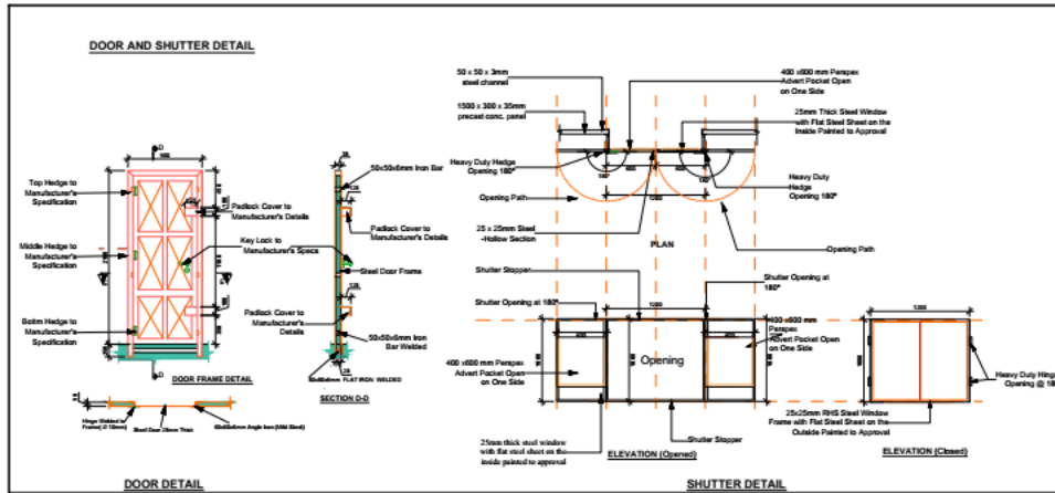
DOOR DETAIL
