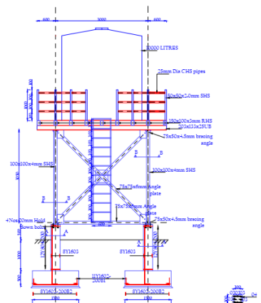
ELEVATION 01
